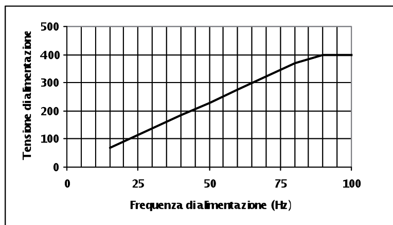
Diag. 4 - Diagramma tensione di alimentazione-frequenza previsto per i motori serie C (230 V / 50 Hz) per il funzionamento a potenza aumentata. Diag. 4 - Supply voltage - frequency diagram intended for the C series motors (230 V / 50 Hz) for operation at increased power.
