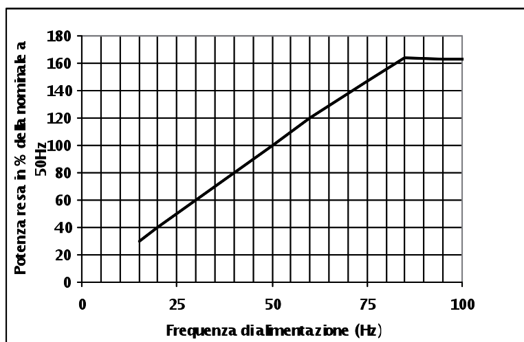
Diag. 5 - Diagramma potenza resa -frequenza per i motori serie CA (220 V / 50 Hz) per il funzionamento a potenza aumentata. Diag. 5 - Power output - frequency diagram intended for the CA series motors (220 V / 50 Hz) for operation at increased power.
