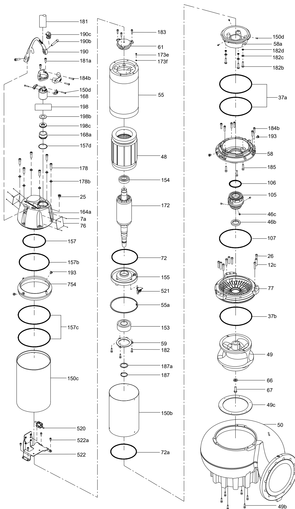
SE2 pumps, 6 poles
